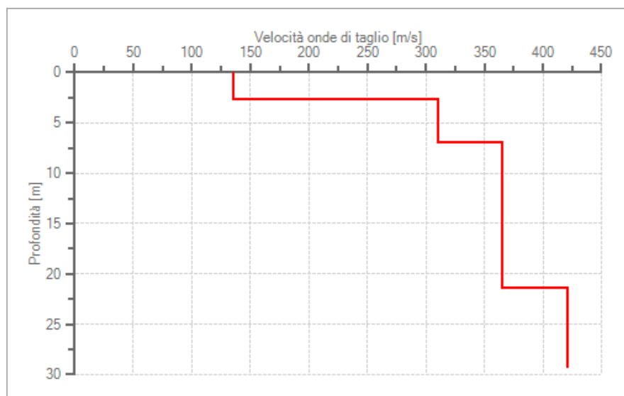
Figura 9 – Profilo Vs da indagine HVSR.
