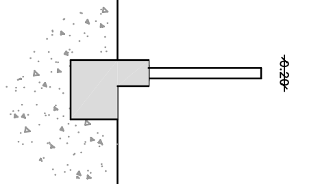
SEZIONE TIPO RECINZIONE Scala 1:50
